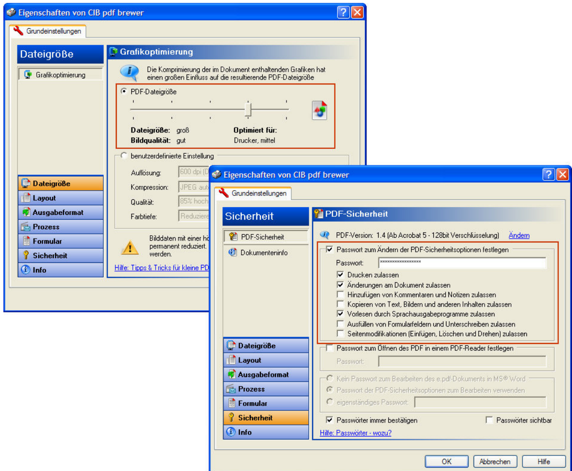
CIB pdf brewer: benutzerfreundlicher Schieberegler zur Reduzierung der PDF-Dateigröße (links); PDF-Sicherheitseinstellungen (rechts)
